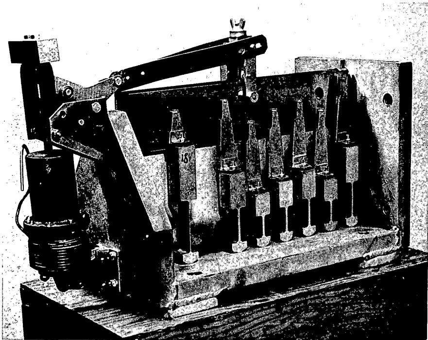
Fig. 10—Shock gauge.
